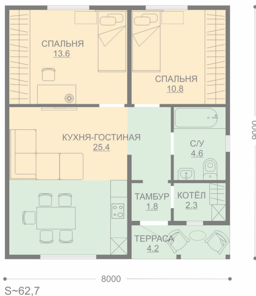
ПЛАН 1-ГО ЭТАЖА
