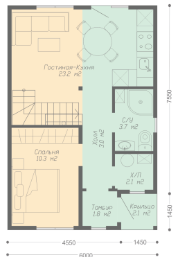
ПЛАН 1-ГО ЭТАЖА
