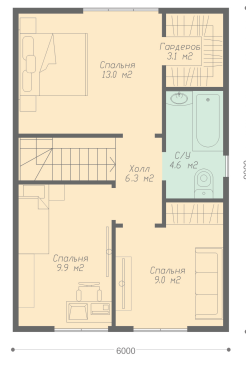
ПЛАН ВТОРОГО ЭТАЖА
