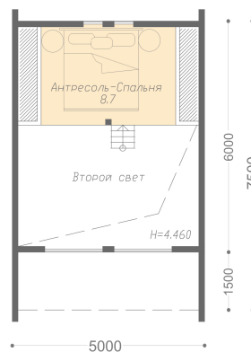
План антресоли
