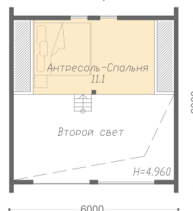
План антресоли
