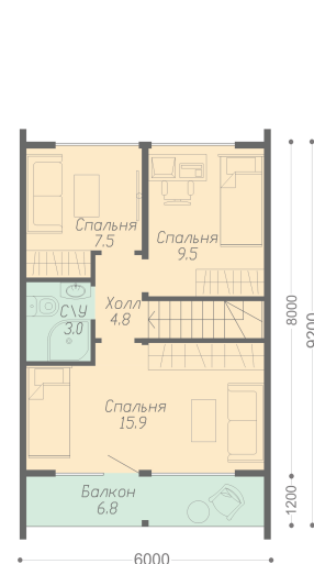
ПЛАН ВТОРОГО ЭТАЖА
