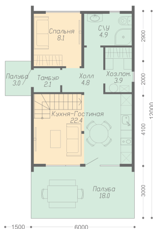
ПЛАН ПЕРВОГО ЭТАЖА
