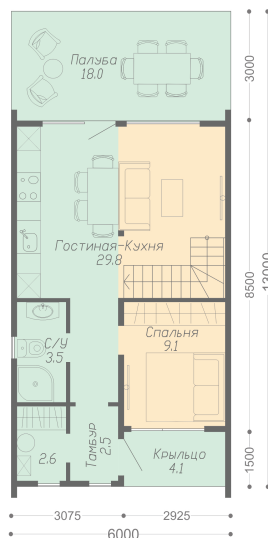
ПЛАН ПЕРВОГО ЭТАЖА
