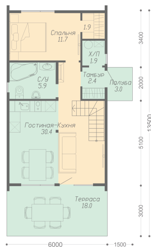
ПЛАН ПЕРВОГО ЭТАЖА
