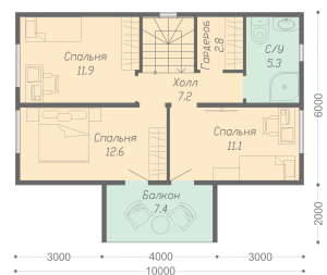
План второго этажа
