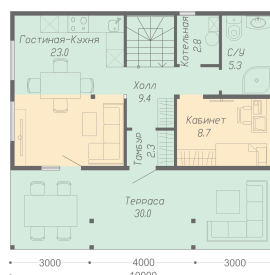
План первого этажа
