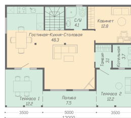
План первого этажа
