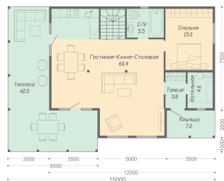
План первого этажа
