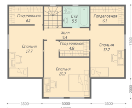
План второго этажа
