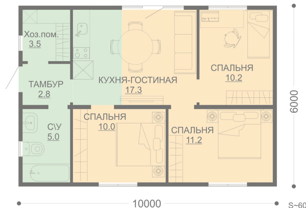
ПЛАН 1-ГО ЭТАЖА
